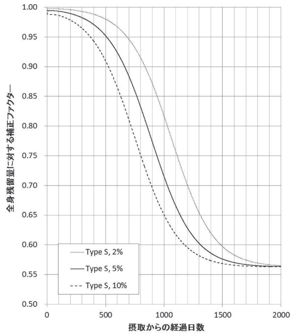
図8 WBC で定量された Cs 全身残留量に対する補正ファクター ※ 137 Cs (AMAD: 5 \mu m) の Type F と Type S の混合摂取の場合
