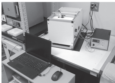
図 2 : ESR 装置の実際
