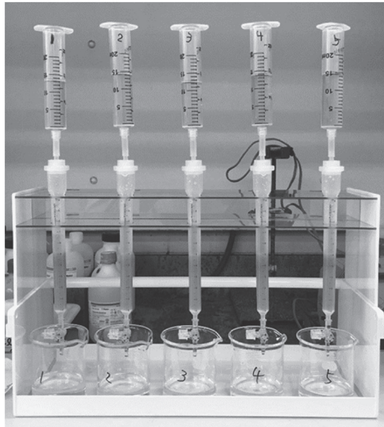
図 11 イオン交換樹脂を用いた尿中ヨウ素分離システム
