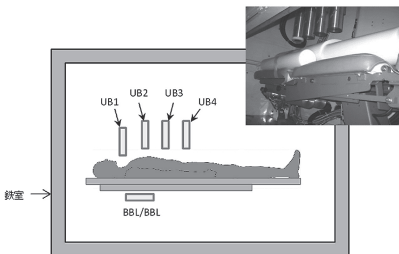
図2 WBCの検出器配置
