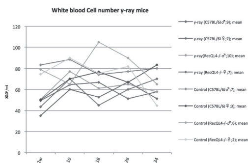
図 19：低線量外部被ばくマウス白血球数変化
