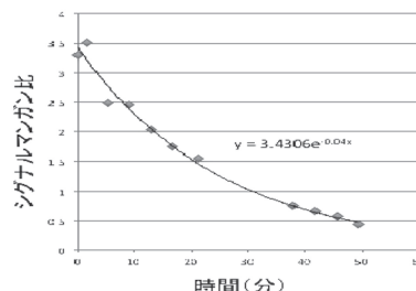
図 4-1 : 全血の還元能 (tempol 還元能)
