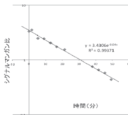
図 4-2 : 全血の還元能 (tempol 還元能)
