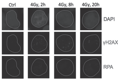
図 11：蛍光免疫染色法による DNA 修復挙動の解析
