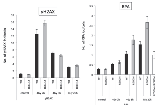
図 12：DNA ダメージ修復タンパク質の挙動の違い (左： \gamma H2AX, 右：RPA)
