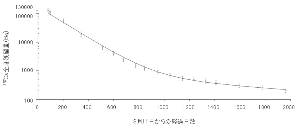
図3 IMBAを用いた解析例 ※実測値（プロット）と予測値（実線）との比較
