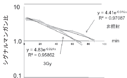
図 7: 放射線照射 14 時間後の細胞内抗酸化力
