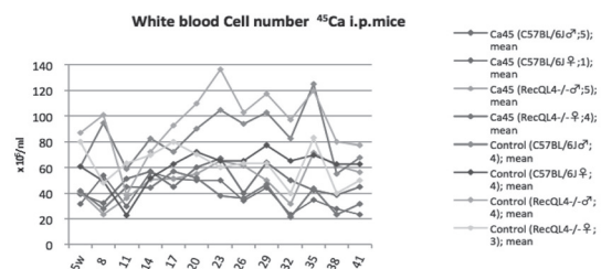
図 16： ^{45}\text{Ca} 注入マウス白血球数変化
