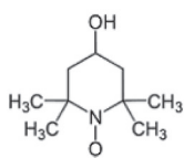
図 1 : tempol 化学構造式
