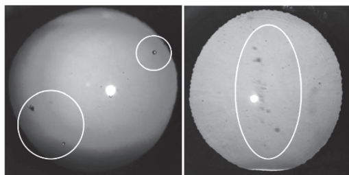
図 1：放射線白内障の初期変化である Vacuoles
