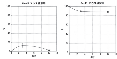
図 13： ^{45}\text{Ca} の排泄率及びマウス残留率
