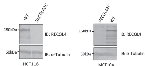
図 9 : Cas9/CRISPR 技術による RecQL4 ノックイン細胞の樹立 (左 : HCT116, 右 : MCF10A)
