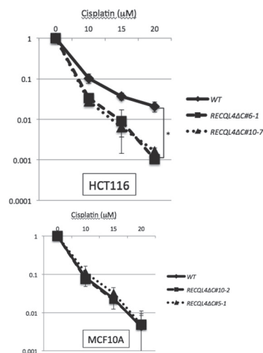
図 10 : シスプラチンに対する感受性の違い (上 : HCT116, 下 : MCF10A)
