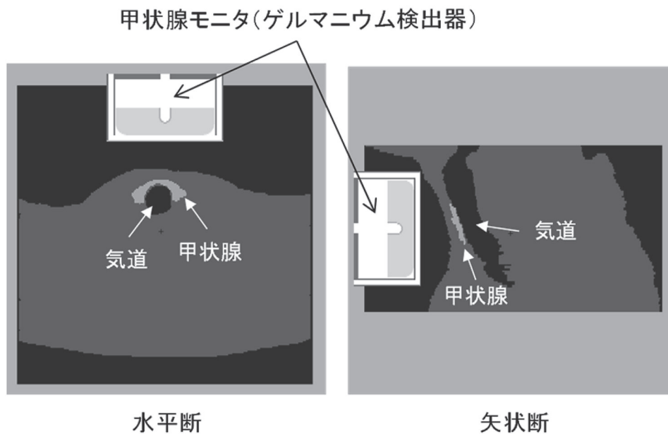
図6 数値シミュレーションのモデル体系
