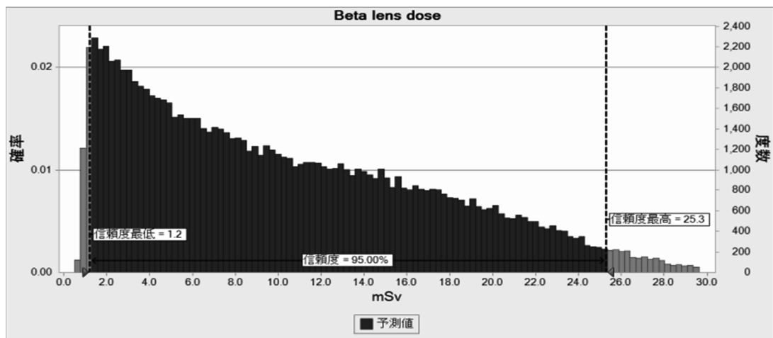
図8 個人線量計の \gamma 線 H_p(10) 指示値 = 100 mSv における \beta 線による水晶体等価線量の分布 (全面マスク着用なし)
