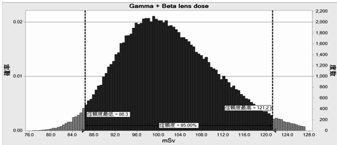
図 10 個人線量計の \gamma 線 H_p(10) 指示値 = 100 mSv における \gamma 線 + \beta 線による水晶体等価線量の分布 (全面マスク着用なし)
