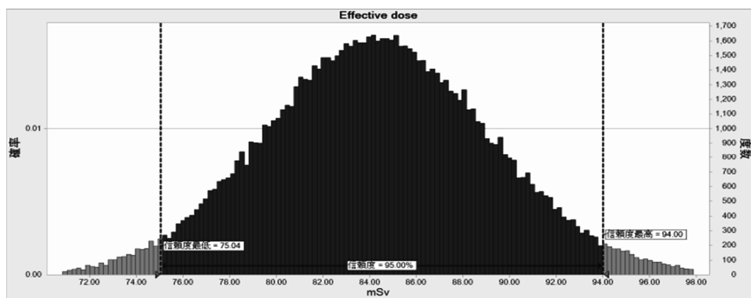
図6 個人線量計の \gamma 線 H_p(10) 指示値=100 mSvにおける \gamma 線実効線量の分布
