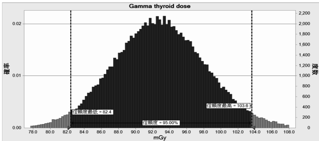
図 12 個人線量計の \gamma 線 H_p(10) 指示値 = 100 mSv における \gamma 線甲状腺吸収線量の分布
