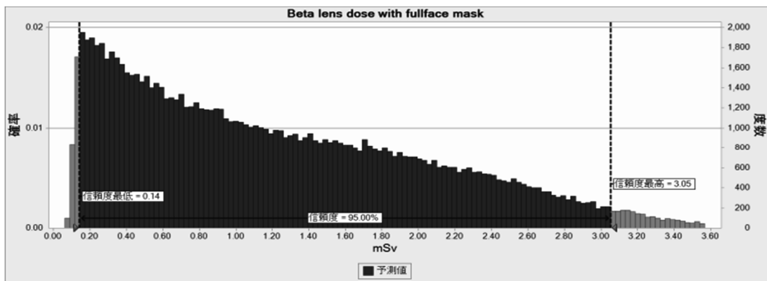
図9 個人線量計の \gamma 線 H_p(10) 指示値 = 100 mSv における \beta 線による水晶体等価線量の分布 (全面マスク着用あり)
