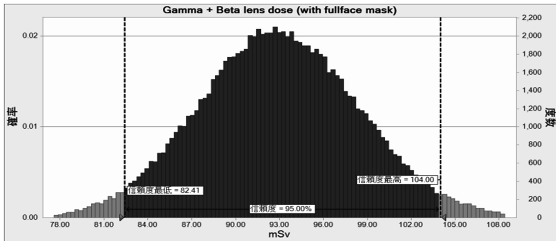
図 11 個人線量計の \gamma 線 H_p(10) 指示値 = 100 mSv における \gamma 線 + \beta 線による水晶体等価線量の分布 (全面マスク着用あり)
