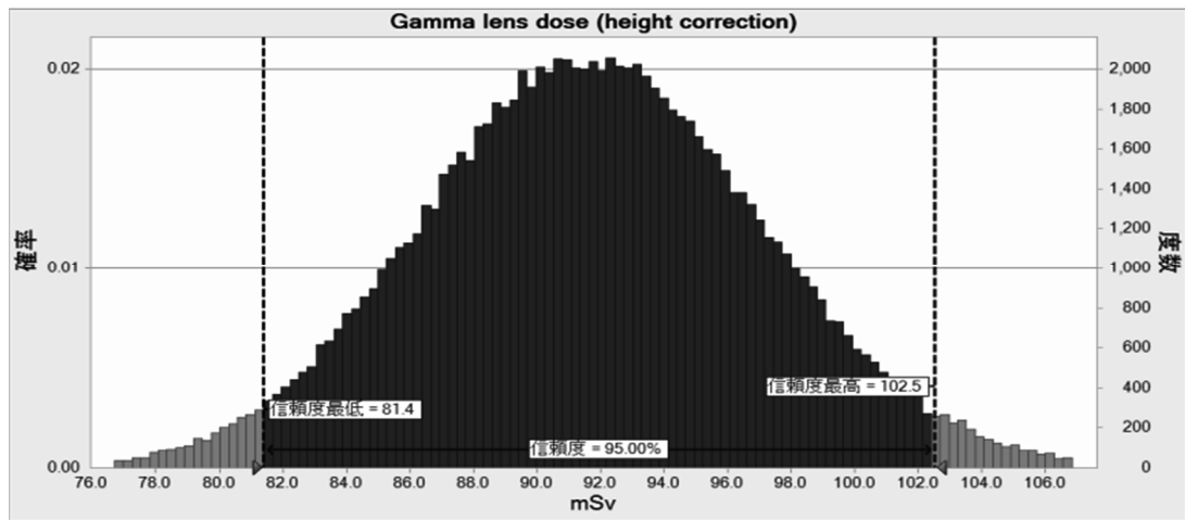
図7 個人線量計の \gamma 線 H_p(10) 指示値 = 100 mSv における \gamma 線による水晶体等価線量の分布 (高さ勾配を補正)
