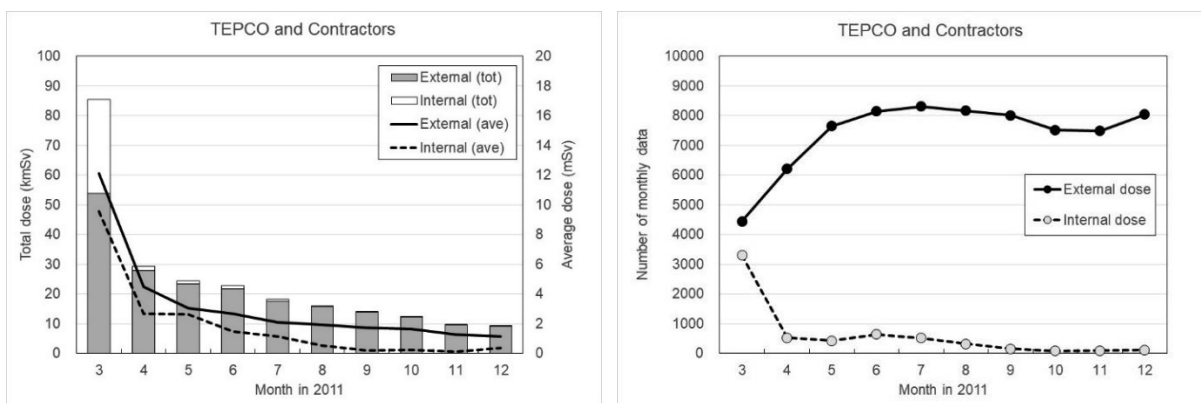
図2 月別線量及び作業件数の推移（東電社員及び協力企業社員） （左は総線量及び平均線量、右は月別データ件数）
